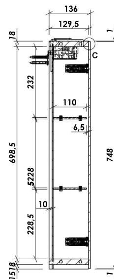
SEZIONE A-A
