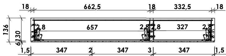
SEZIONE B-B
