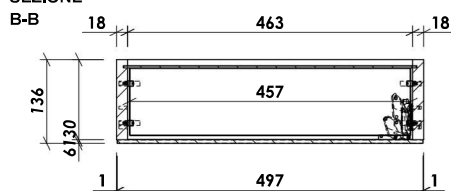
SEZIONE B-B
