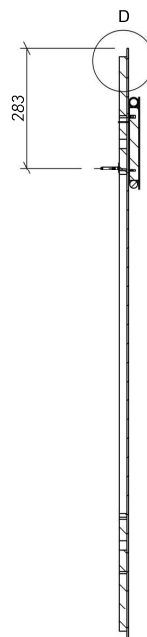
SEZIONE C-C
